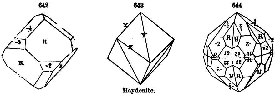
Haydenite.
